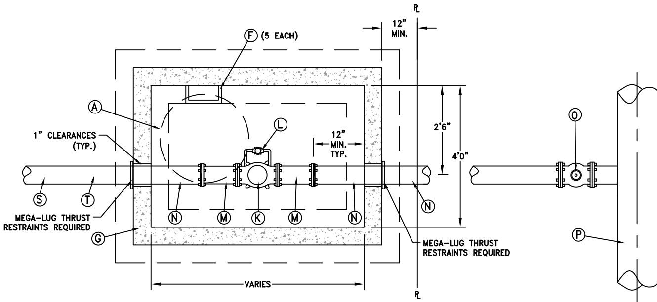
PLAN N.T.S.
