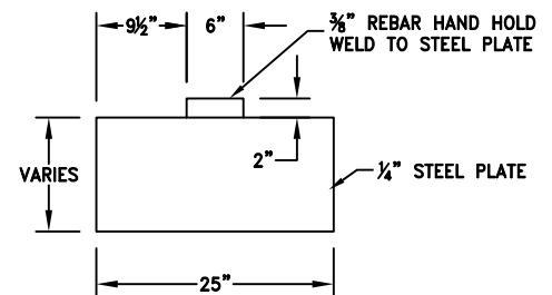
GATE DETAIL N.T.S.
