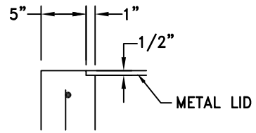
CONCRETE NOTCH N.T.S.
