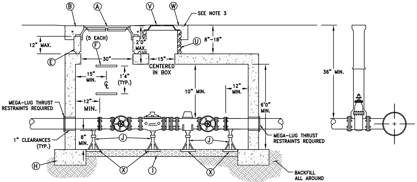
ELEVATION N.T.S.
