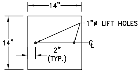
LID DETAIL N.T.S.
