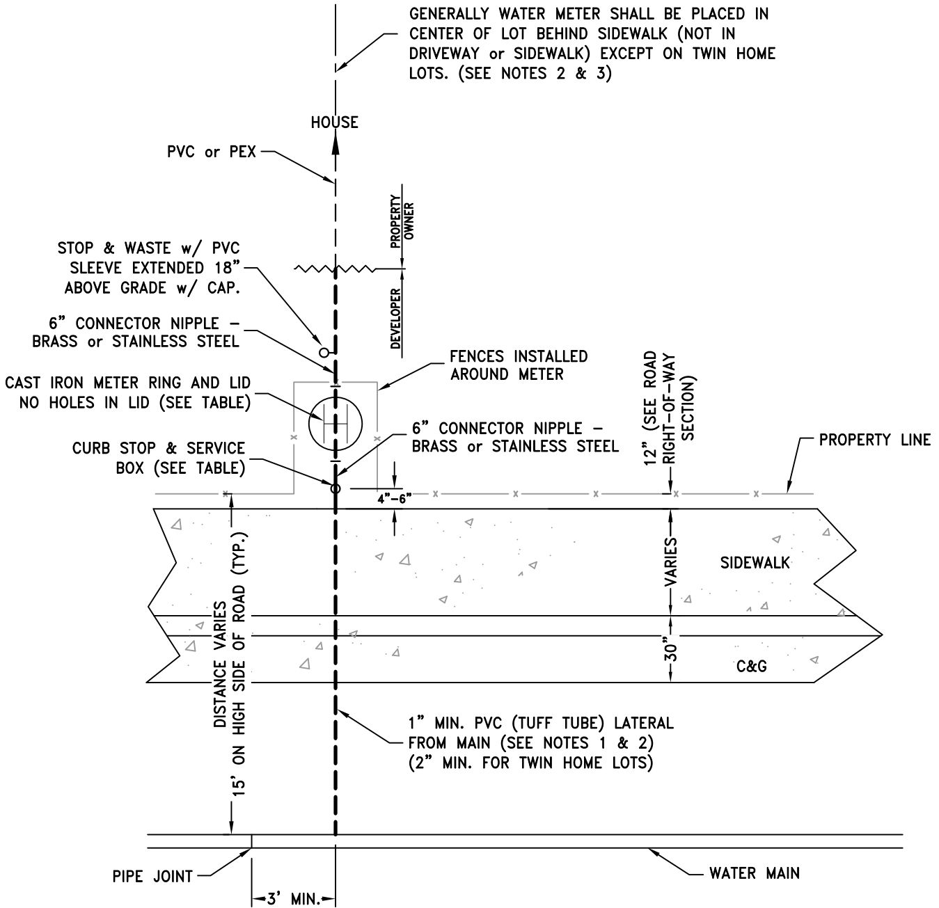
PLAN N.T.S.
