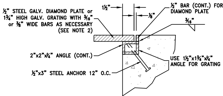
ANCHOR DETAIL N.T.S.
