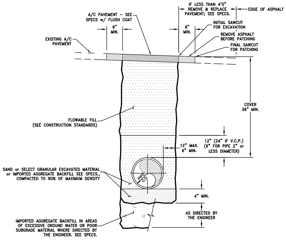
TYPICAL TRENCH DETAIL N.T.S.
