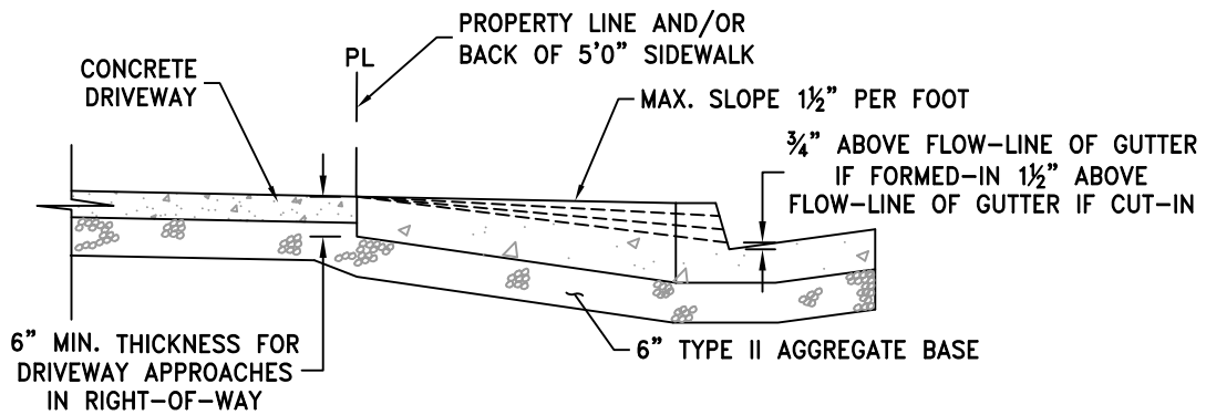
SECTION N.T.S.
