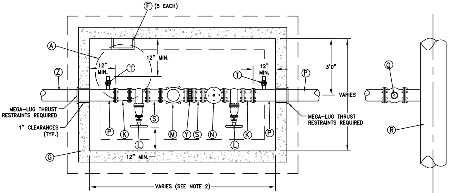
PLAN N.T.S.
