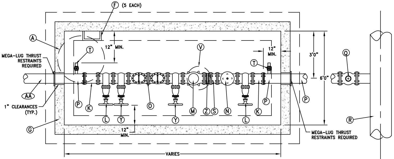
PLAN N.T.S.
