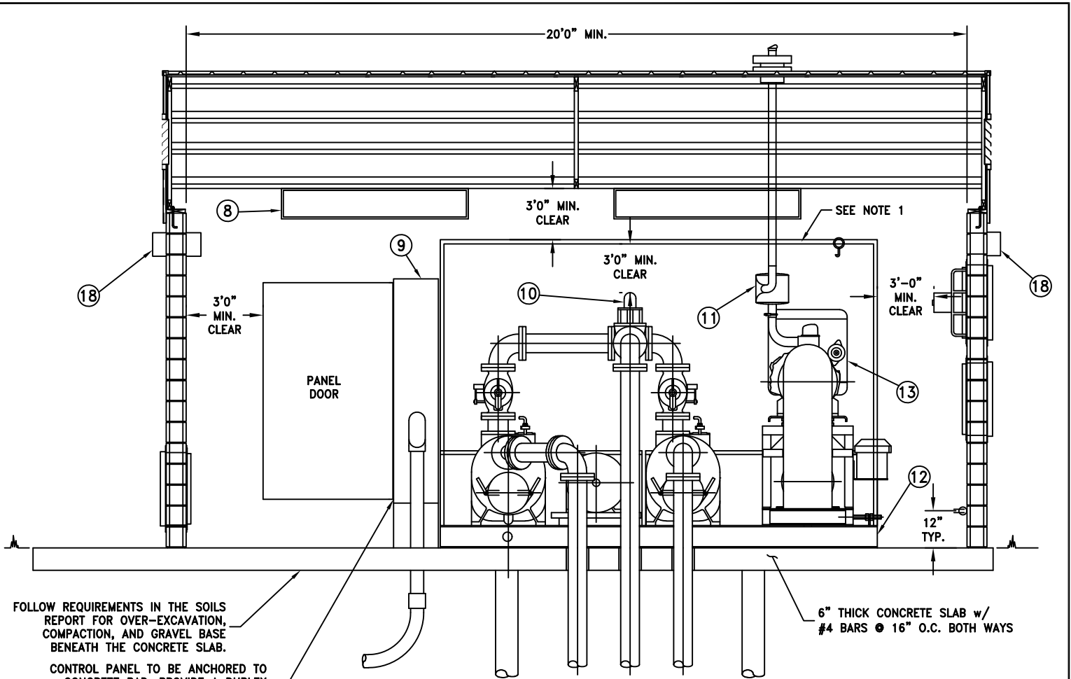
PUMP FRONT ELEVATION N.T.S.
