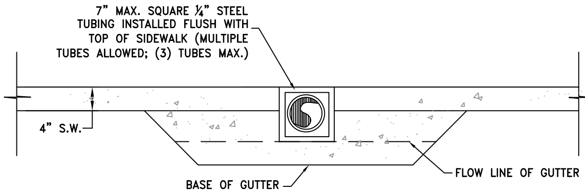
SECTION N.T.S.
