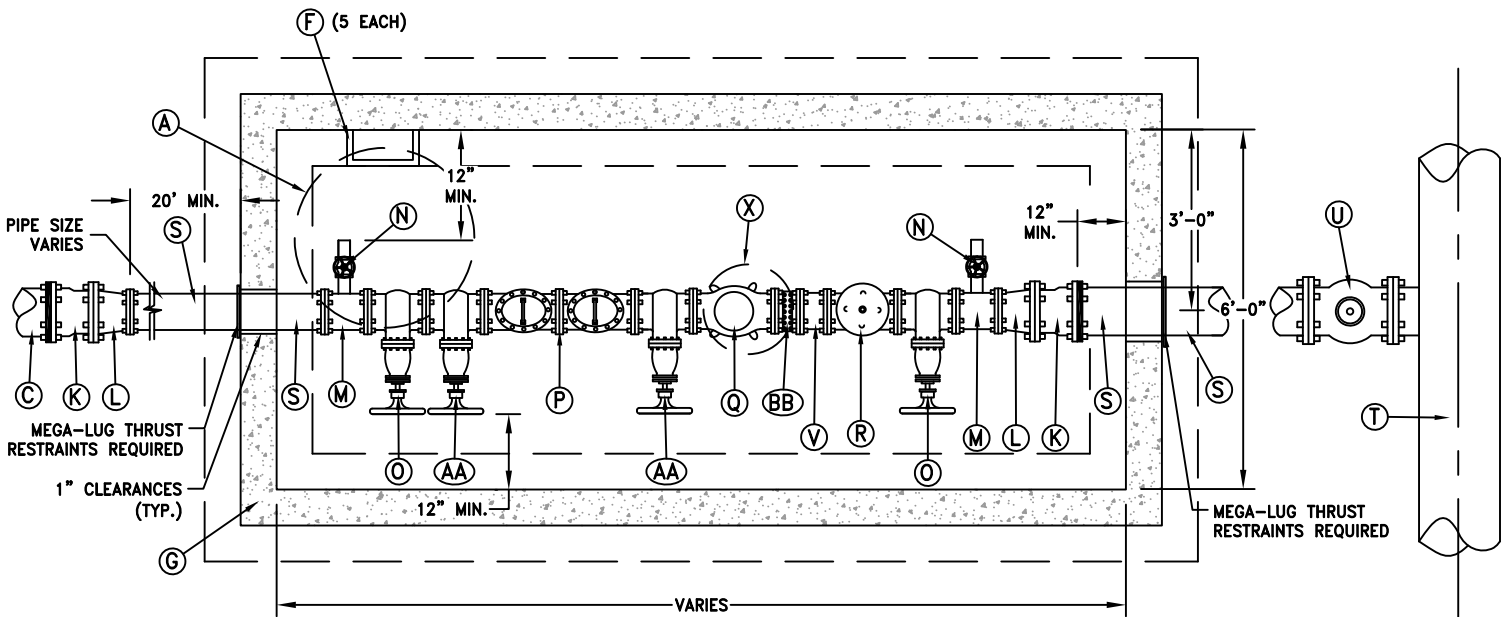
PLAN N.T.S.
