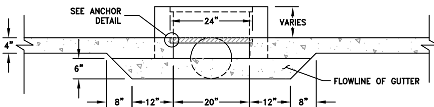
SECTION C-C N.T.S.
