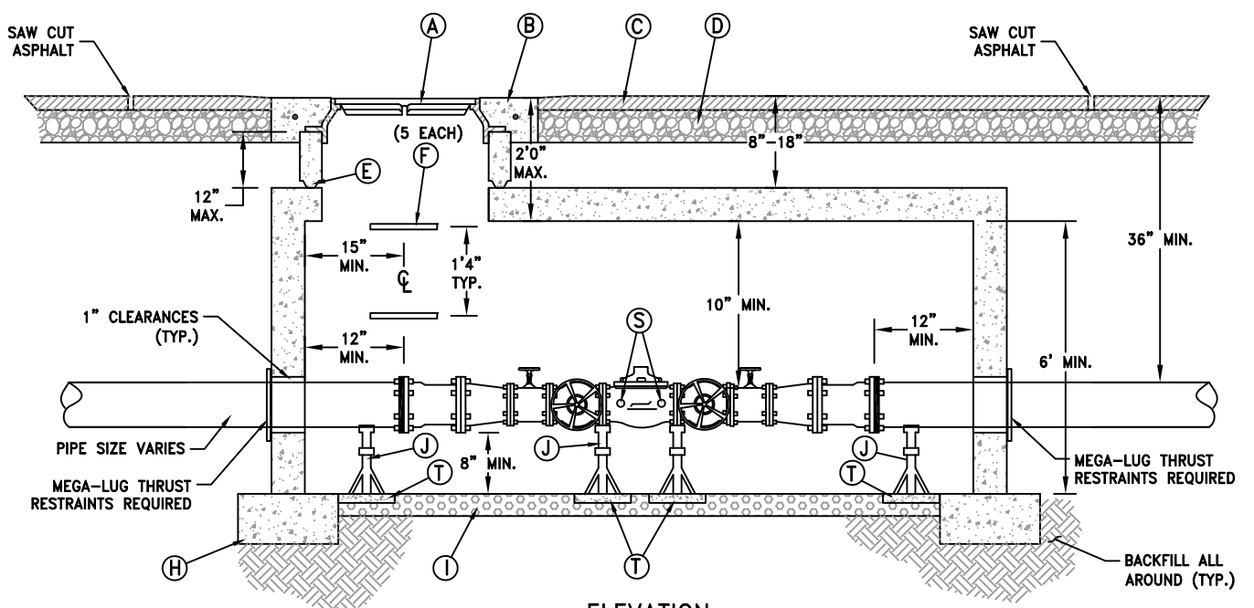
ELEVATION N.T.S.
