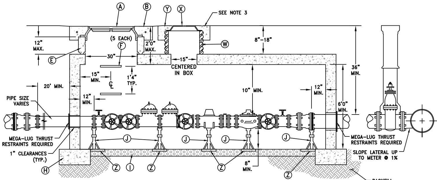
ELEVATION N.T.S.
