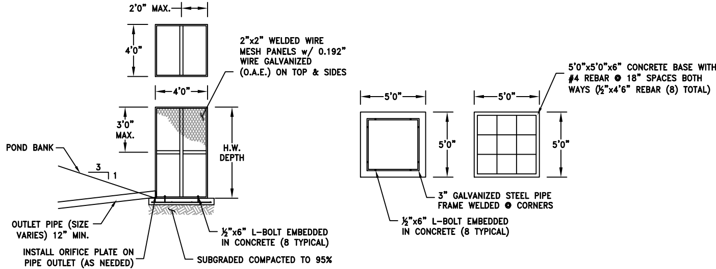
SCREEN POND OUTLET DETAIL N.T.S.
