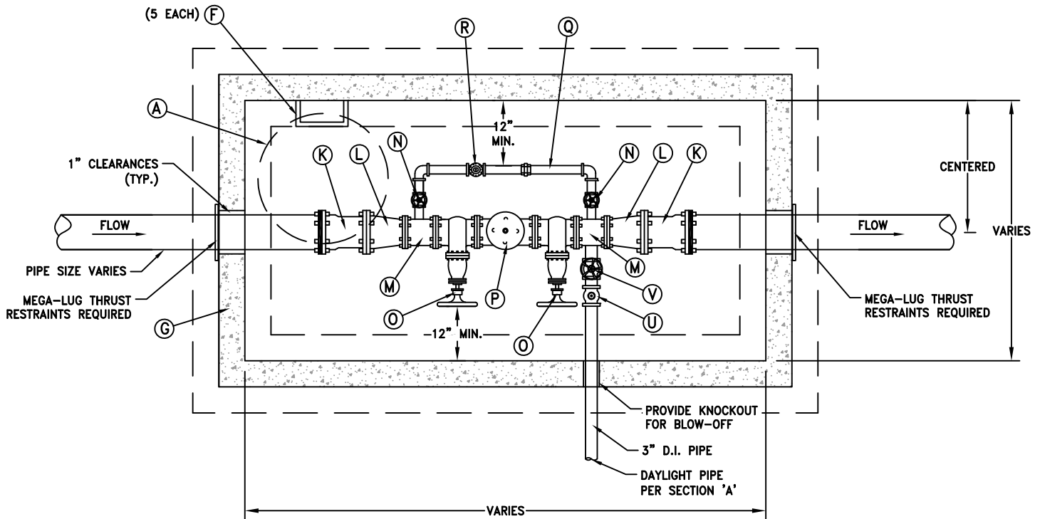
PLAN N.T.S.
