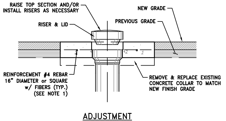
VALVE COLLAR DETAIL N.T.S.
