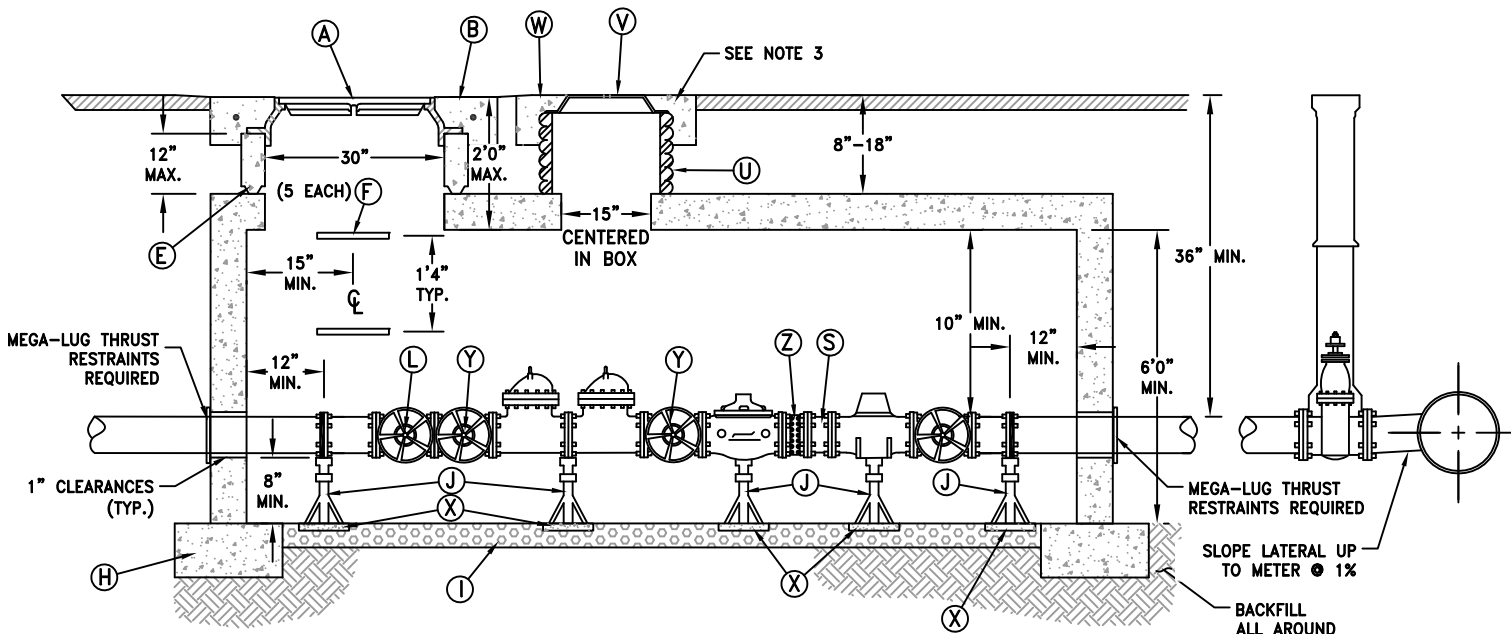
ELEVATION N.T.S.
