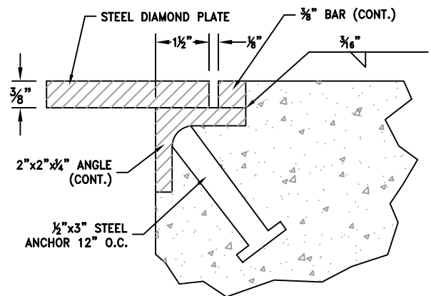
ANCHOR DETAIL N.T.S.
