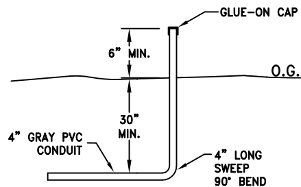
DETAIL 'A'- SPARE CONDUIT VERTICAL LOCATE RISER N.T.S.
