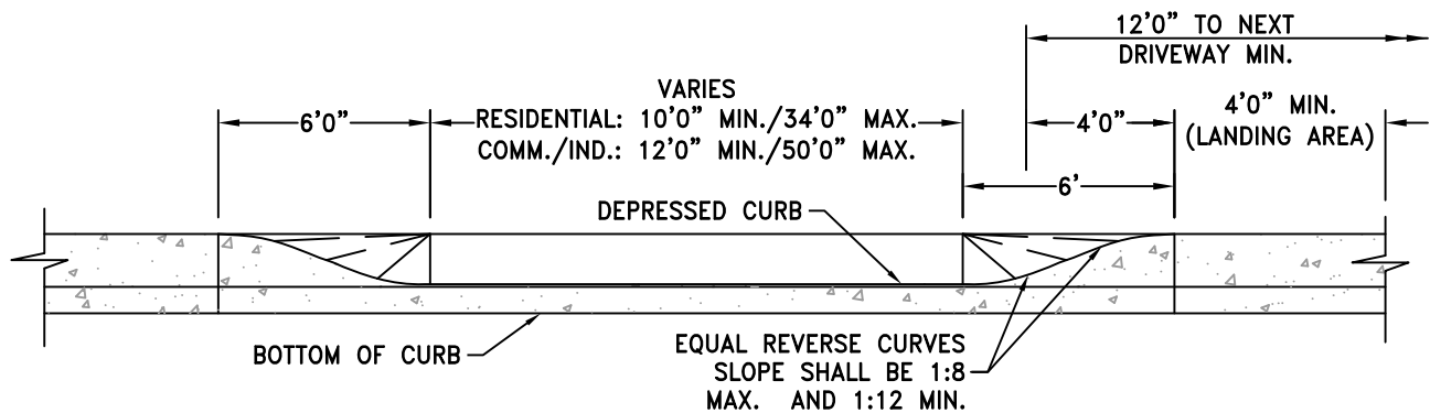
ELEVATION N.T.S.
